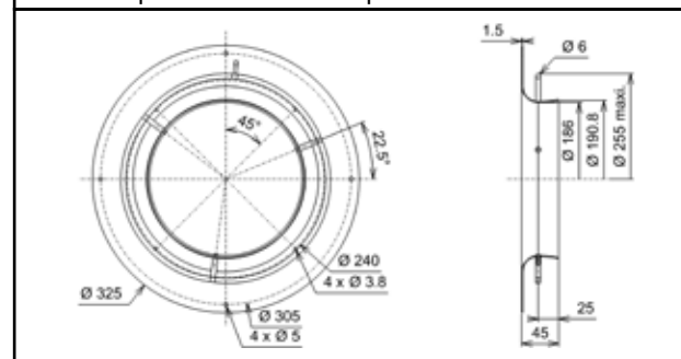
16284 pour turbine / for impeller / für Laufrad Ø280
