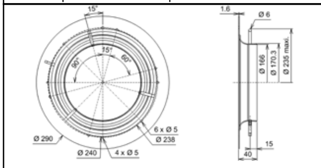
16283 pour turbine / for impeller / für Laufrad Ø250
